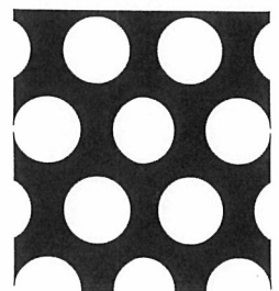
8φ×12P 開孔率(約40%)
