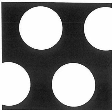
20φ×30P 開孔率(約40%)
